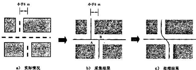
图11 相同方向道路中心线之间的距离小于5 m时,应相交于同一点
