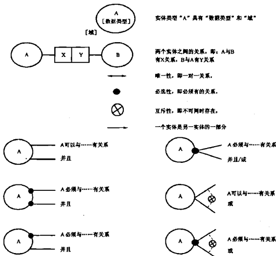
图1 NIAM模型表达符号
