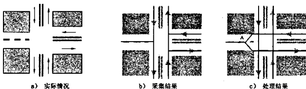
图9 物理隔离带在路口处断开
