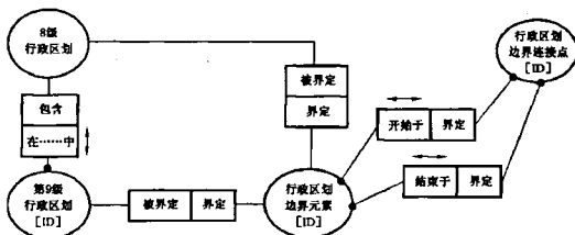
图 23 行政区划 1-层要素数据模型
