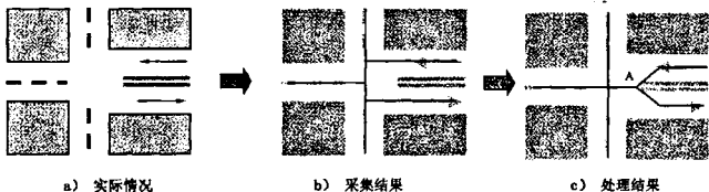
图7 物理隔离带在路口之前断开
