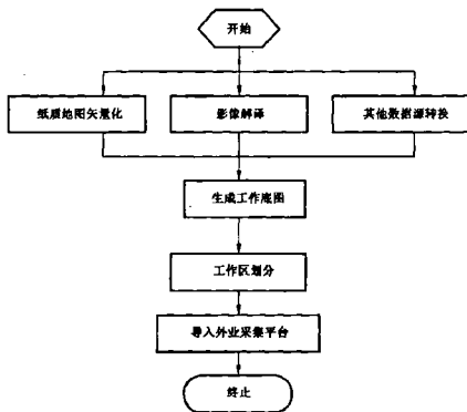
图4 数据预处理流程
