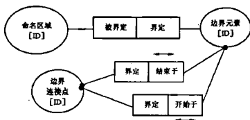
图24 命名区域 1-层要素数据模型
