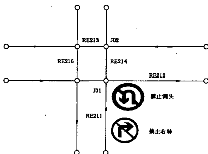
图 44 禁止规则
