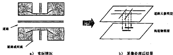
图 27 以多个线要素表示的构造物
