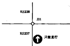
图 45 限制规则
