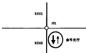
图 43 优先规则
