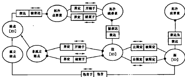
图 2 完全拓扑的定义
