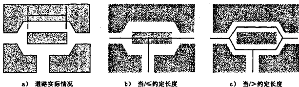
图 18 丁字路口矩形交通岛处理要求
